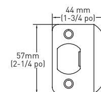
GÂCHE À COINS ARRONDIS AVEC LANGUETTE PLEINE LARGEUR
